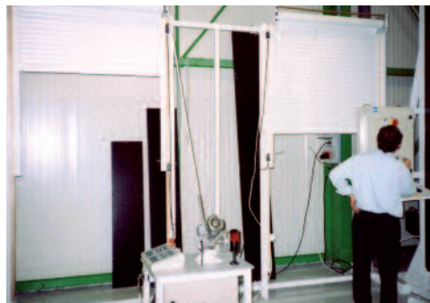
Banc d'Essais au Vent de Volet Roulant (BVV)
