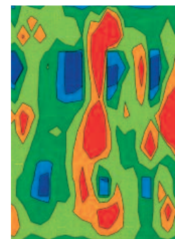
Cartographie des vides sous un dallage (zones rouges)
